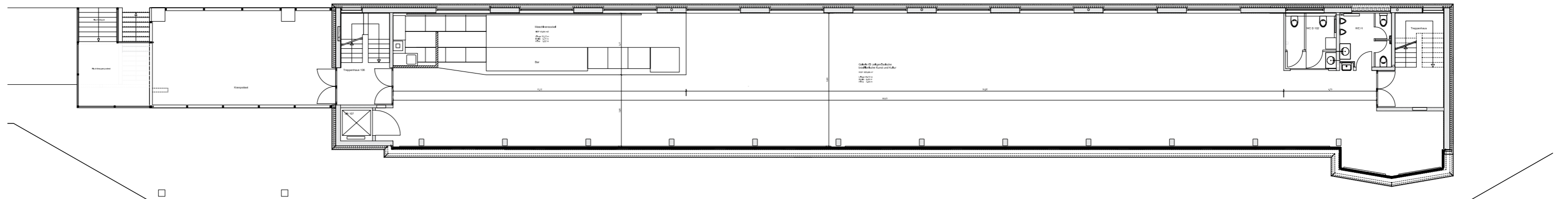
HOCHPARTERRE 350 m 2 max. 420 Personen 1:200 L 50.72 m B 6.84 m H 3.69 m
