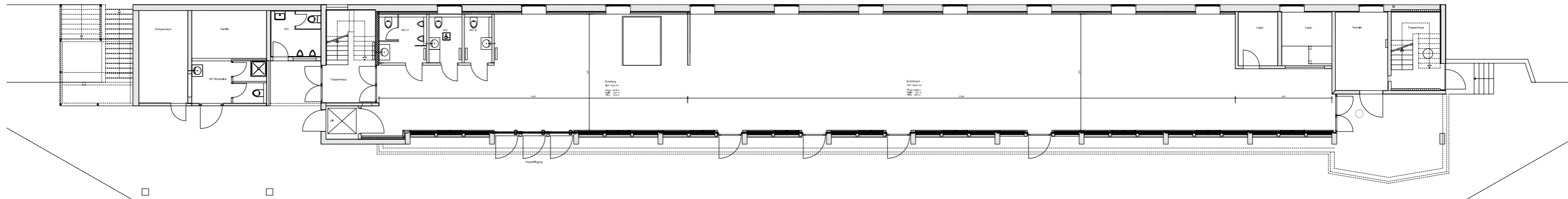
SOCKELGESCHOSS 260 m 2 max. 350 Personen 1:200 L 43.70 m B 5.91 m H 3.25 m
